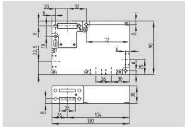
Schmersal. Соленоидная блокировка — EX-AZM 161SK-12/12K-024-3D
