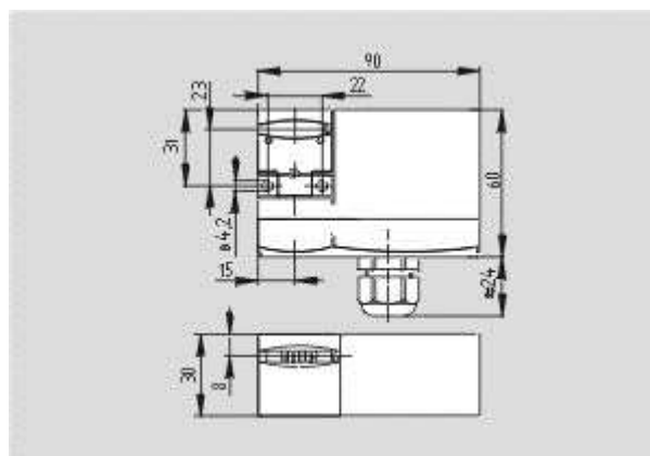
Schmersal. Соленоидная блокировка — EX-AZM 170-02ZRKA-24VAC/DC-3G/D
