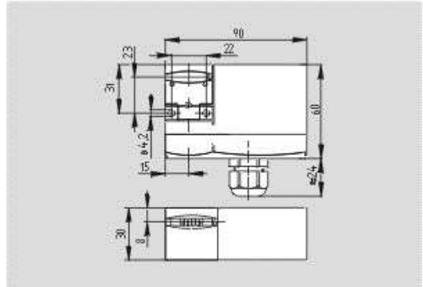
Schmersal. Соленоидная блокировка — EX-AZM 170-02ZK-24VAC/DC-3G/D
