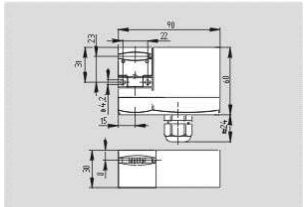
Schmersal. Соленоидная блокировка — EX-AZM 170-11ZRK 24VAC/DC-3G/D
