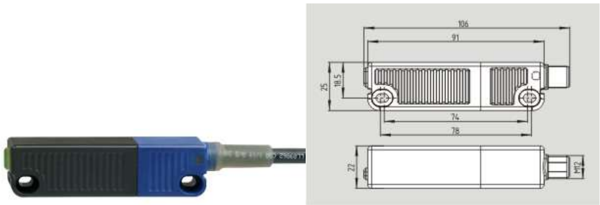
Schmersal. Датчики безопасности — RSS 36-11-D-R
