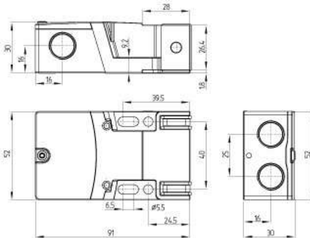
Schmersal. Датчики безопасности — RSS16-I2-D-CC
