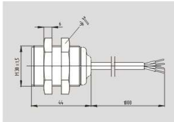
Schmersal. Датчики безопасности — BNS 303-12Z 3,0M
