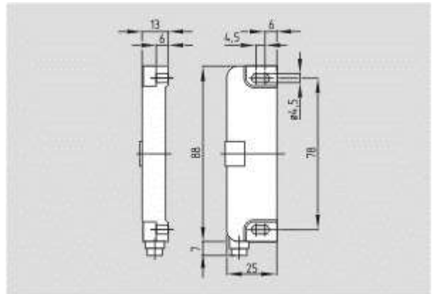
Schmersal. Датчики безопасности — BNS 36-02/01Z-ST-L
