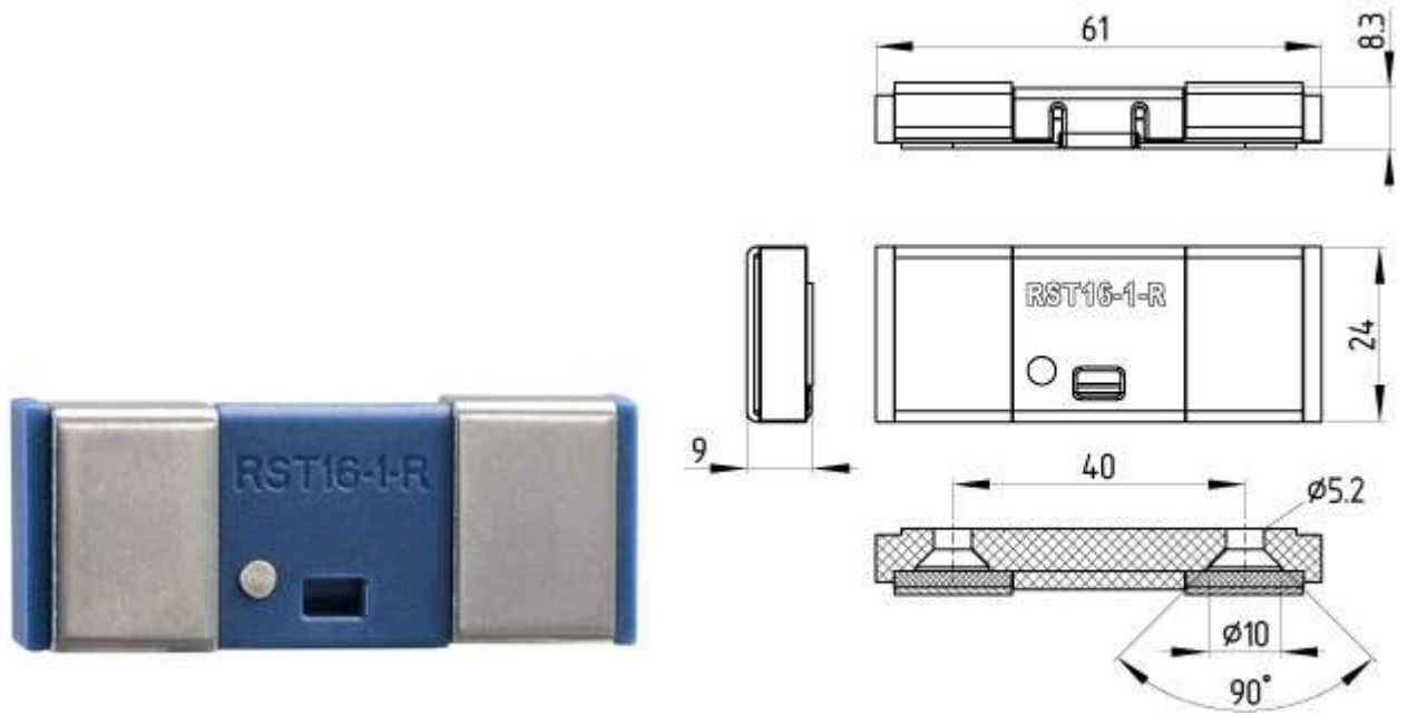
Schmersal. Датчики безопасности — RST16-1-R
