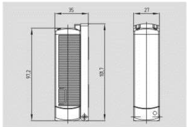
Schmersal. Датчики безопасности — BNS 16-12ZU-ST1
