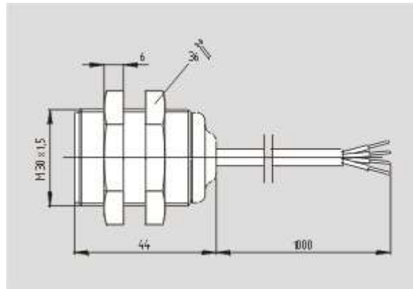
Schmersal. Датчики безопасности — BNS 303-11Z 10,0M
