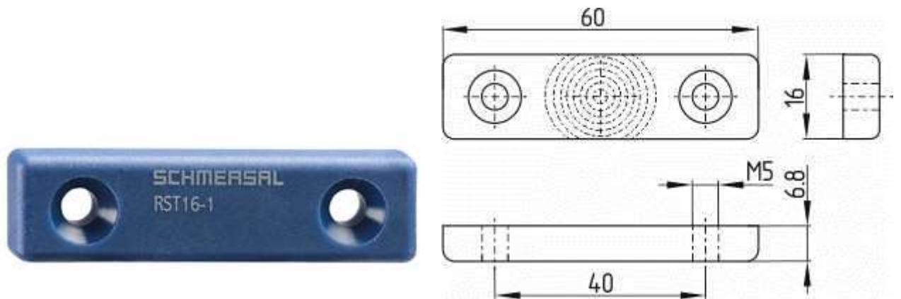
Schmersal. Датчики безопасности — RST16-1
