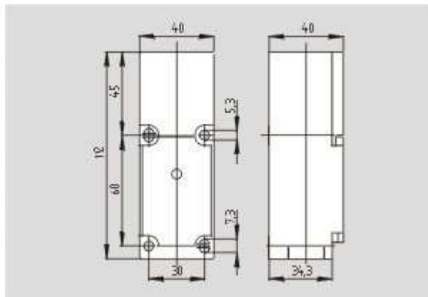
Schmersal. Датчики безопасности — BNS 333-01yU
