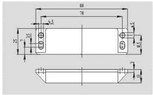
Schmersal. Датчики безопасности — BPS 33-2326
