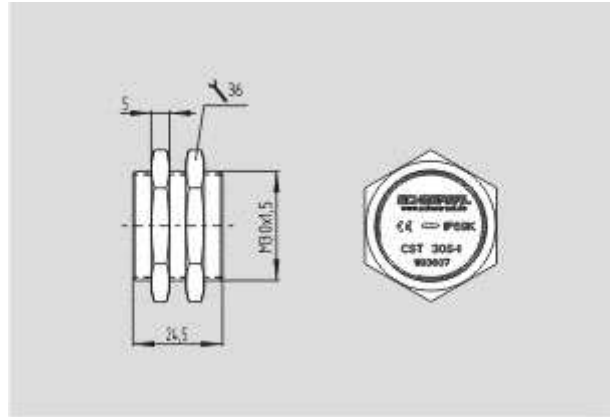
Schmersal. Датчики безопасности — CST 30S-1
