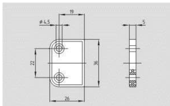
Schmersal. Датчики безопасности — SPACER BNS 260
