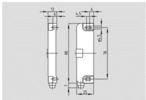
Schmersal. Датчики безопасности — BNS 36-02/01ZG-ST-R
