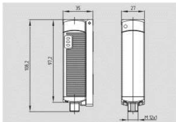
Schmersal. Датчики безопасности — CSS 12-34-V-SD-M-L
