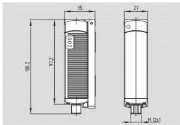
Schmersal. Датчики безопасности — CSS 14-34-S-SD-M-L
