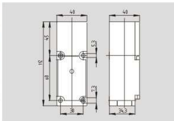
Schmersal. Датчики безопасности — BNS 333-01yD
