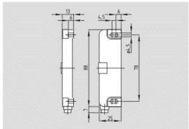
Schmersal. Датчики безопасности — BNS 36-11/01Z-ST-L
