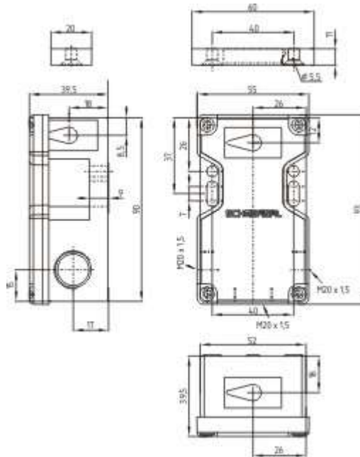
Schmersal. Датчики безопасности — BNS 16-12ZU-ST1
